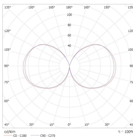
KANLUX S.A. (kat 38418) XLED C35E14 7W-CW / Krzywa rozsyłu światła (biegunowo)
