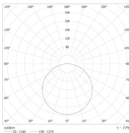
KANLUX S.A. (kat 37305) IPER LED 35W-NW-L-SE / Krzywa rozsyłu światła (biegunowo)
