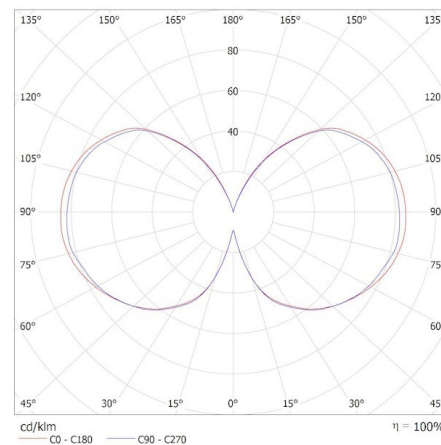
KANLUX S.A. (kat 37240) XLEDIM A60 E27 11W-WW / Krzywa rozsyłu światła (biegunowo)
