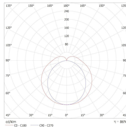
KANLUX S.A. (kat 36667) AKVO IP44 23W-NW-C / Krzywa rozsyłu światła (biegunowo)
