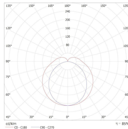
KANLUX S.A. (kat 36662) AKVO IP44 20W-NW-W / Krzywa rozsyłu światła (biegunowo)
