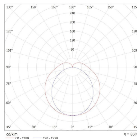
KANLUX S.A. (kat 36658) AKVO IP44 23W-NW-C S / Krzywa rozsyłu światła (biegunowo)
