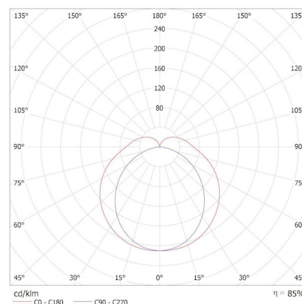
KANLUX S.A. (kat 36653) AKVO IP44 20W-NW-W S / Krzywa rozsyłu światła (biegunowo)
