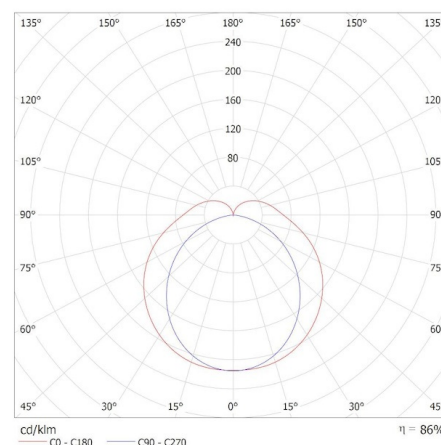
KANLUX S.A. (kat 36652) AKVO IP44 15W-NW-C S / Krzywa rozsyłu światła (biegunowo)
