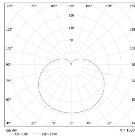
KANLUX S.A. (kat 33721) IQ-LED A60 13,5W-CW / LDC (Polar)
