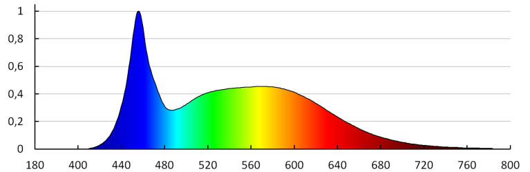
KANLUX S.A. (kat 33721) IQ-LED A60 13,5W-CW / LDC (Polar)
