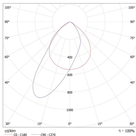
KANLUX S.A. (kat 33477) FL AGORIA HI 240W NW / LDC (Polar)
