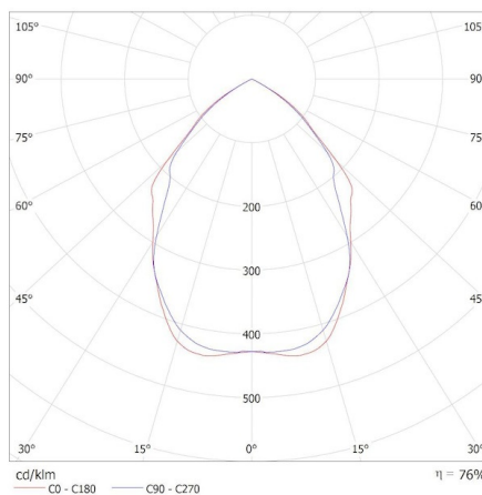
KANLUX S.A. (kat 33139) ATL2 GU10-B + IQ-LED ... 6,5WS3 / Krzywa rozsyłu światła (biegunowo)
