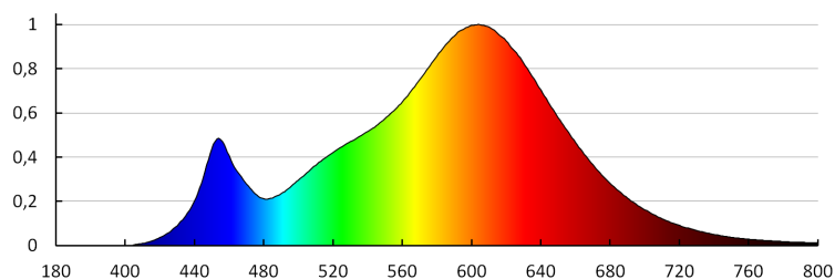
MILED o (kat 31233) GU10 6W-WW LED / LDC (Polar)
