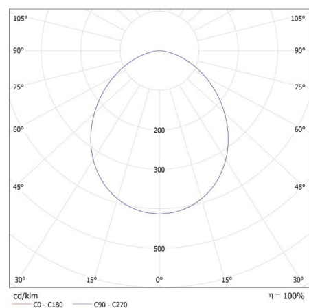
MILED o (kat 31233) GU10 6W-WW LED / LDC (Polar)
