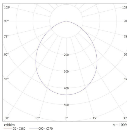
MILEDO (kat 31227) GU10 2,7W-WW LED / Krzywa rozsyłu światła (biegunowo)
