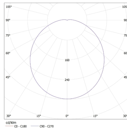
MILEDO (kat 31091) DUNO LED N15W-NW-O / LDC (Polar)
