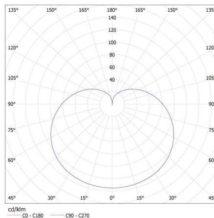
KANLUX S.A. (kat 27314 IQ-LED A67 17,5W-CW / LDC (Polar)
