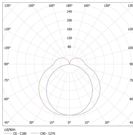
KANLUX S.A. (kat 27115) TP SLIM LED 40W-NW / LDC (Polar)
