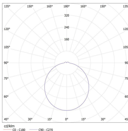
KANLUX S.A. (kat 26986) VARSO HI 36W-NW-L-SE / LDC (Polar)
