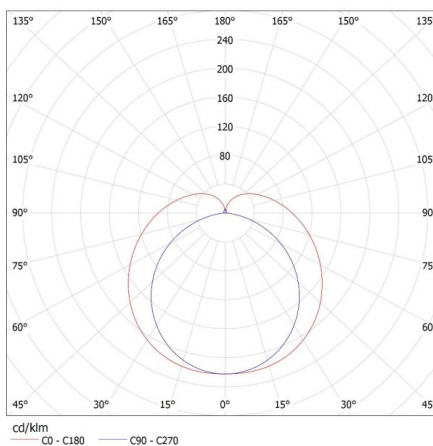
KANLUX S.A. (kat 26700) ROLSO LED IP44 15W-NW / Krzywa rozsyłu światła (biegunowo)
