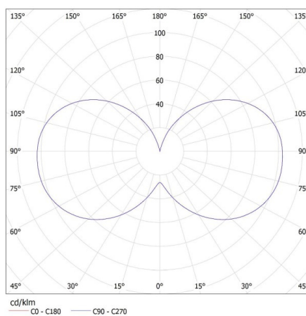
KANLUX S.A. (kat 24524) ZUBI HI LED4WG9-WW / Krzywa rozsyłu światła (biegunowo)
