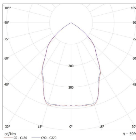
KANLUX S.A. (kat 18192) GORDO N 1W CW-L-SR / LDC (Polar)
