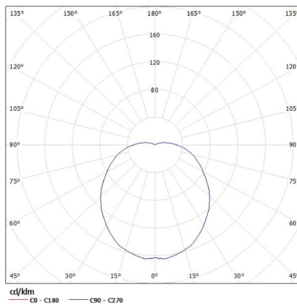
KANLUX S.A. (kat 18120) FOGLER DL-240O / Krzywa rozsyłu światła (biegunowo)
