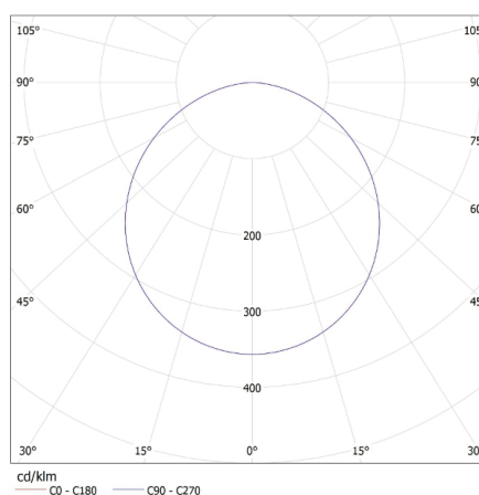
MILEDO (kat 31083) SP LED N 18W NW-R / LDC (Polar)
