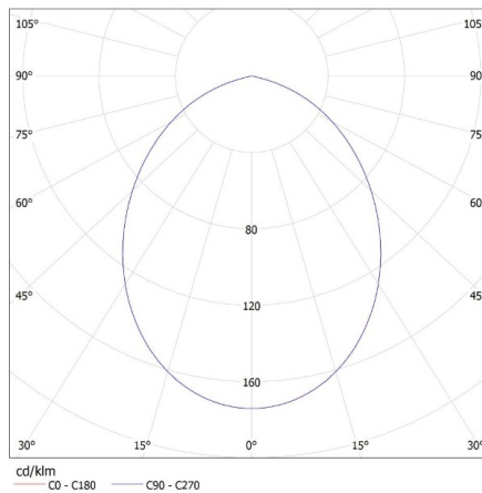
KANLUX S.A. (kat 24362) SONOR GU10 CO-B + TOMI / LDC (Polar)
