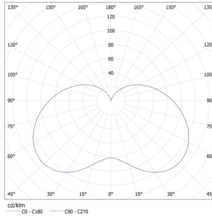
KANLUX S.A. (kat 23382) IDO 4,5W T SMD E14-WW / Krzywa rozsyłu światła (biegunowo)
