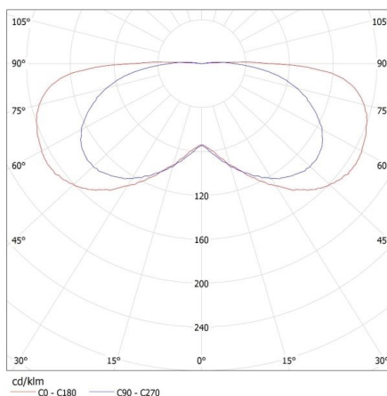
KANLUX S.A. (kat 23105) TERRA MINI LED / Krzywa rozsyłu światła (biegunowo)
