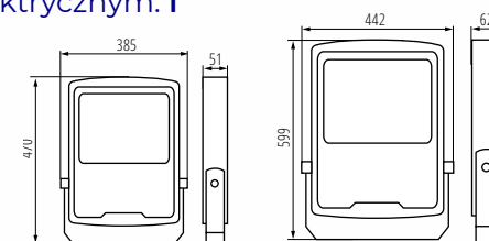
FL AGOR HI 240W FL AGOR-A HI 240W
